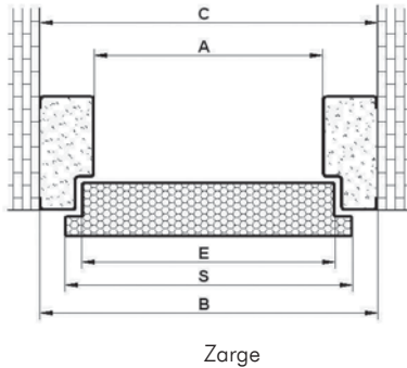
ASYMMETRISCHE PORTALZARGE MIT DICHTUNG FR (für Türen WD, WDT, WP 30, WP 30 (S), S, C, CT)
