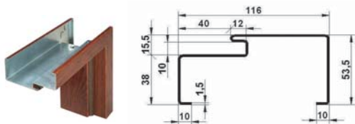
ASYMMETRISCHE ZARGE MIT DICHTUNG FA SL (für Türen APX 3010D, WX 10, CX 10, SX 10, WX 20, CX 20, SX 20, GSX, GWX 20)
