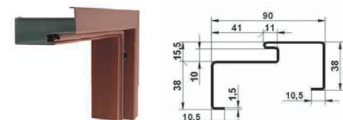
ASSYMETRISCHE ZARGE MIT DICHTUNG FA (für Türen TT PLUS, TT MAX, GTT PLUS, GTT MAX)
