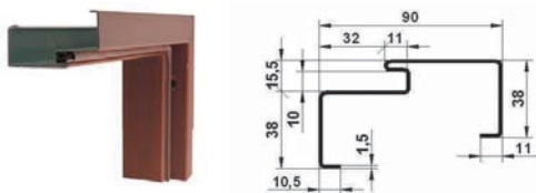
ASSYMETRISCHE ZARGE MIT DICHTUNG FA (für Türen TT, GTT)
